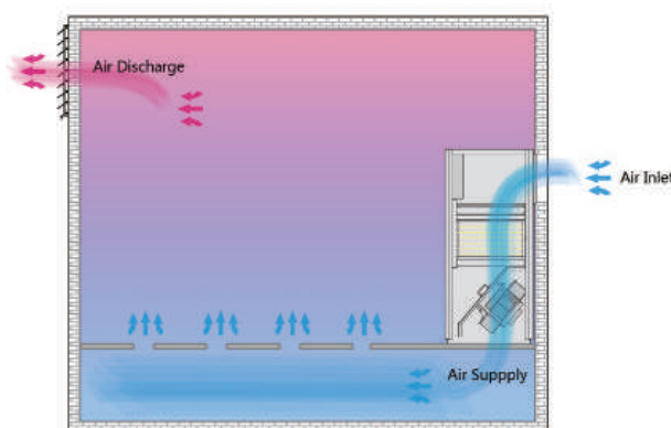
Schema Luftführung durch das Gerät Version U - unten ausblasend
